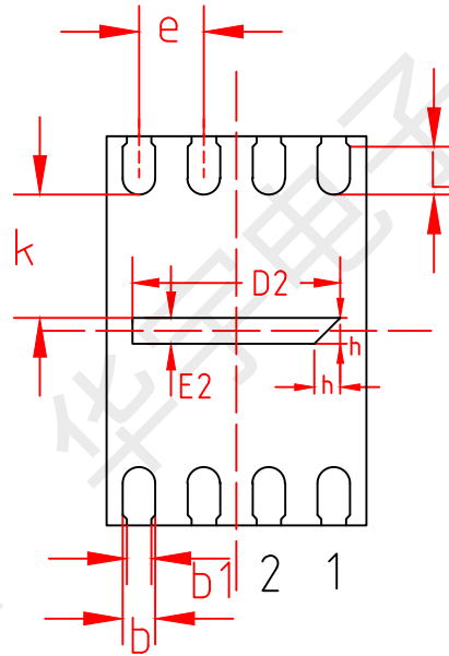
BOTTOM VIEW 背视图
