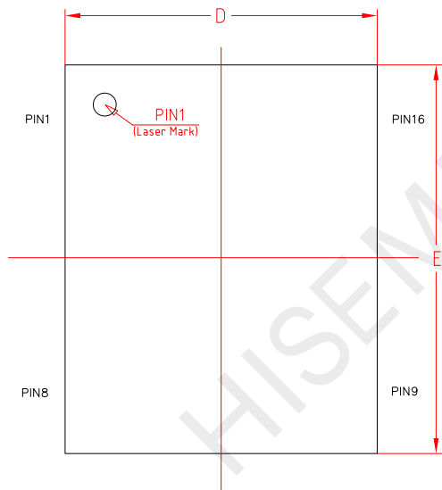
正视图
