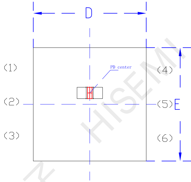
TOP VIEW 正视图
